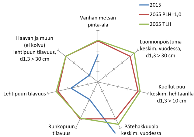
c) Pohjois-Suomi: Taso70 PLH vs. Taso70 TLH
