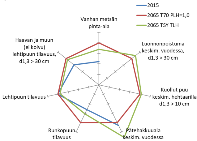
b) Etelä-Suomi: Taso70 PLH vs. TasoSY TLH
