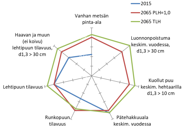
b) Etelä-Suomi: Taso70 PLH vs. Taso70 TLH
