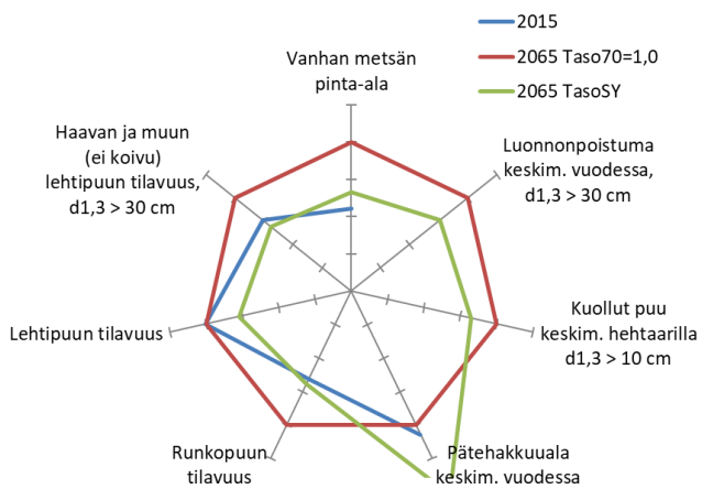
b) Etelä-Suomi: Taso70 PLH vs. TasoSY PLH
