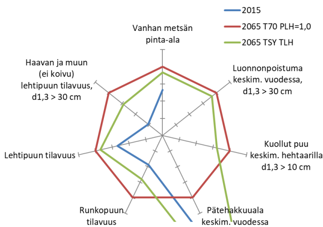
c) Pohjois-Suomi: Taso70 PLH vs. TasoSY TLH
