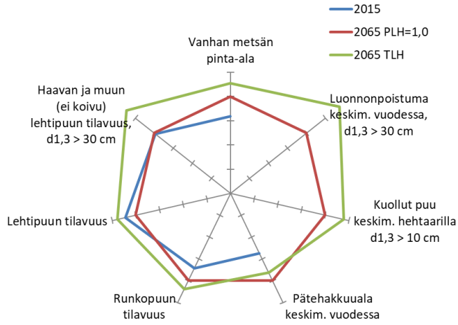
a) Suomi: TasoSY PLH vs. TasoSY TLH
