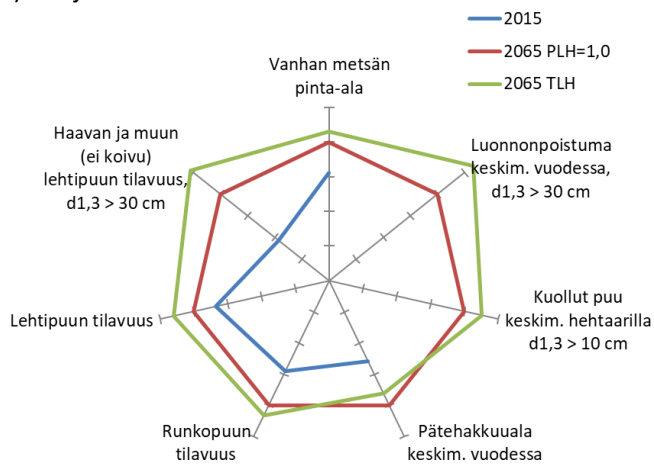
c) Pohjois-Suomi: TasoSY PLH vs. TasoSY TLH
