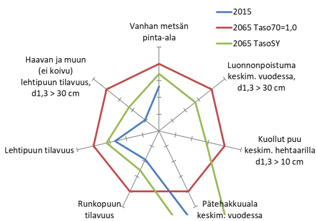
c) Pohjois-Suomi: Taso70 PLH vs. TasoSY PLH
