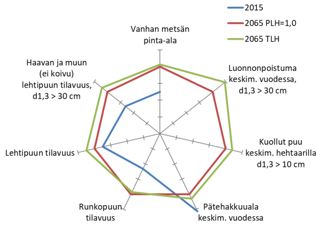
a) Suomi: Taso70 PLH vs. Taso70 TLH
