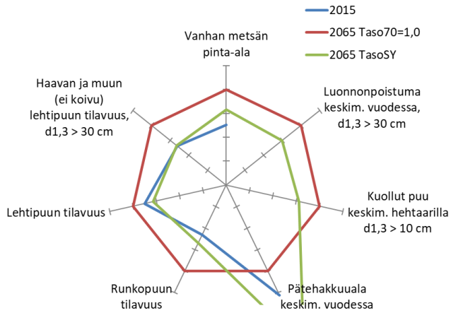
a) Suomi: Taso70 PLH vs. TasoSY PLH
