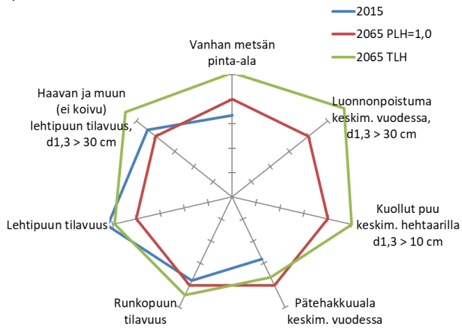
b) Etelä-Suomi: TasoSY PLH vs. TasoSY TLH
