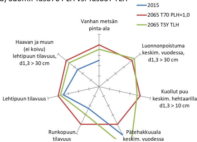
a) Suomi: Taso70 PLH vs. TasoSY TLH
