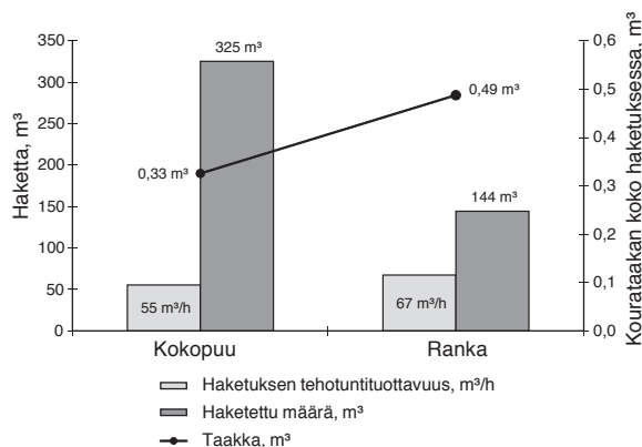
Kuva 6. Kokopuun ja rangan haketuksen tehontuntuottavuus kiintokuutiometreinä (m 3 /h), taakkakoon keskiarvo haketuksessa (m 3 ) sekä aikatutkimuksissa haketettu puumäärä (m 3 ).
