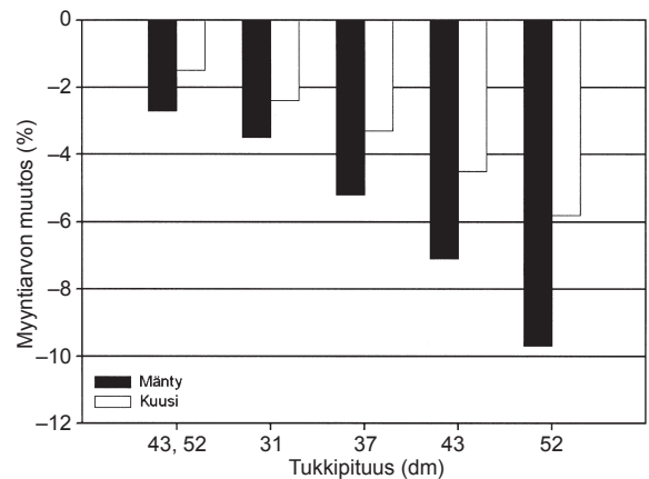
Kuva 5. Männen ja kuusen myyntiarvojen muutokset yhdellä tukkipituudella sekä pituuksilla 43 ja 52 dm. Tukin minimiläpimittana oli männällä 15 cm ja kuusella 16 cm. Vertailutasona on apteeraus pituuksilla 40–55 dm.
