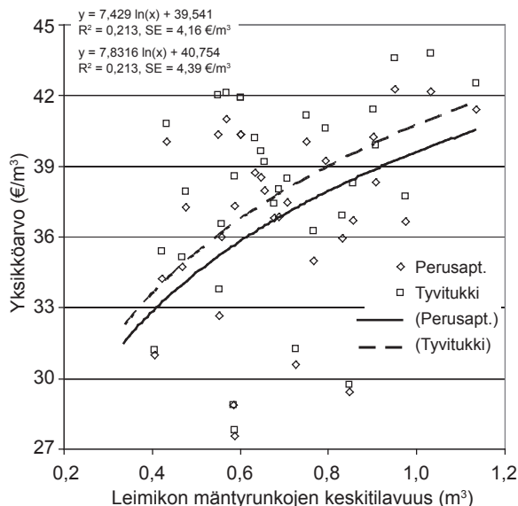
Kuva 9. Keskijäreyden vaikutus männyn simuloituihin ja malleilla ennustettuihin yksikköarvoihin perus- ja tyvitukkiapteerauksessa. Aineistona Metsäliiton leimikot, joissa oli tukkipuun mittavaatimukset täyttäviä mäntyjä (32 leimikkoa).
