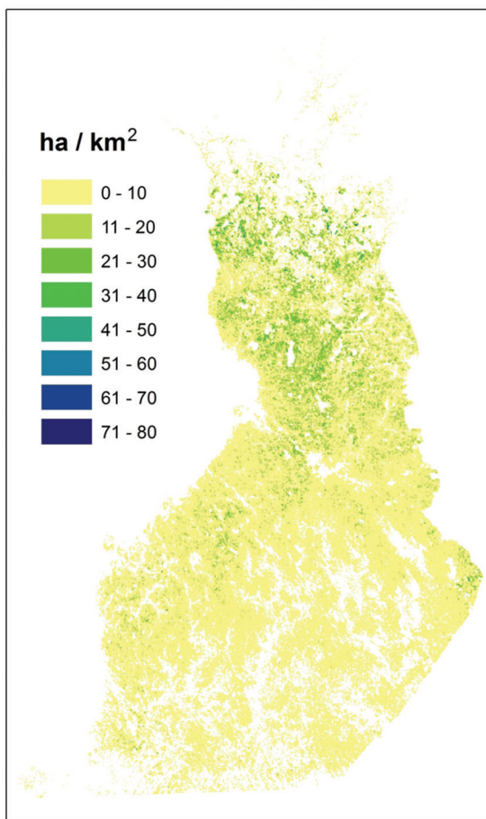
Kuva 4. Monilähdeinventoinnin kartta-aineiston käsittelyssä kitu- tai joutomaaksi määritettyjen kuvioiden kokonaispinta-ala yhden neliökilometrin ruuduissa. (Huom. Yksittäisten heikkotuottoisten suokuvioiden karttamuotoinen esittäminen koko maan mittakaavassa ei ole käytännössä mahdollista.)
