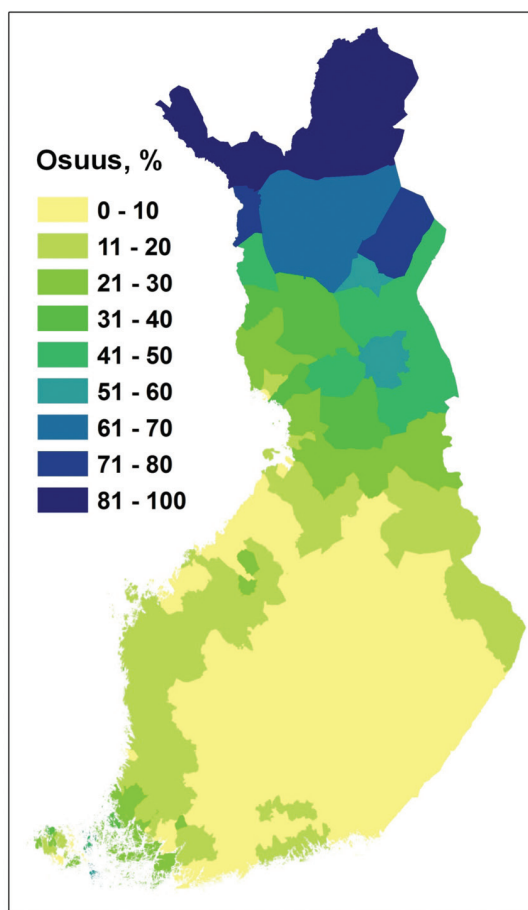
Kuva 5. Monilähdeinventoinnin kartta-aineiston käsittelyssä kitu- tai joutomaaksi määritettyjen kuvioiden osuus vuoden 2011 kuntien metsäojitettujen soiden kokonaispinta-alasta. Myös ojitetujen soiden kokonaispinta-ala perustuu monilähdeinventointiin.
