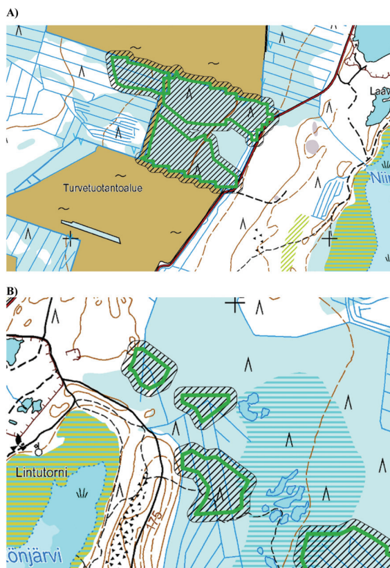
Kuva 1. A) Heikkotuottoisten kuvioiden (vihreä viiva) etäisyys on lyhimmillään alle 50 m, ja niiden ympärille luodut vyöhykkeet (musta vinoviivitus) muodostavat spatiaalisesti jatkuvan polygonin: laskennassa samaa kuviota. B) Heikkotuottoisten kuvioiden etäisyys on lyhimmillään yli 50 m, ja niiden ympärille luodut vyöhykkeet eivät kosketa toisiaan: laskennassa jokainen kuvio on erillinen.
